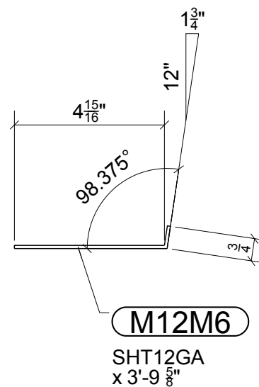
ONE - PAN - M12M6
