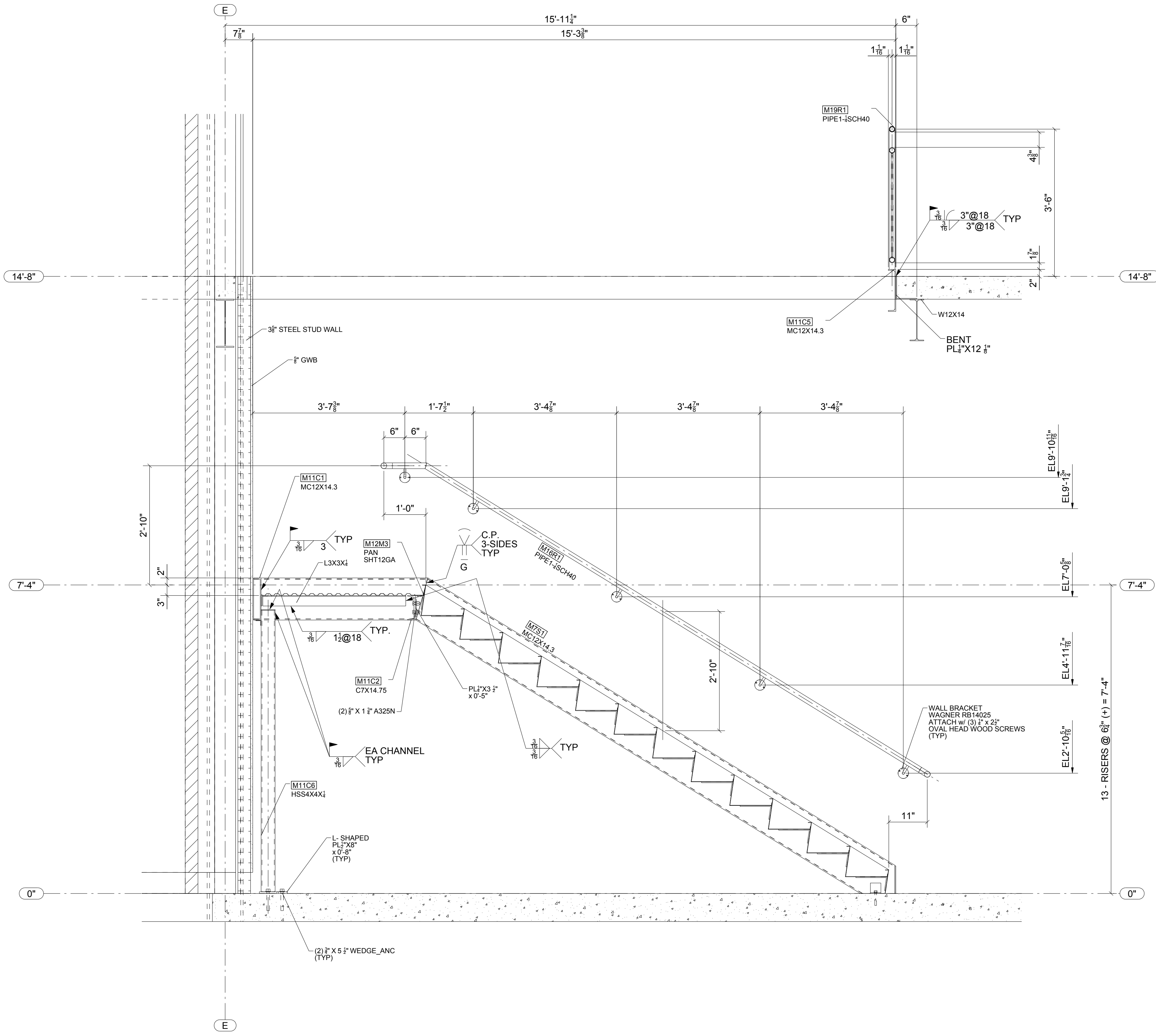
B - B ME1
