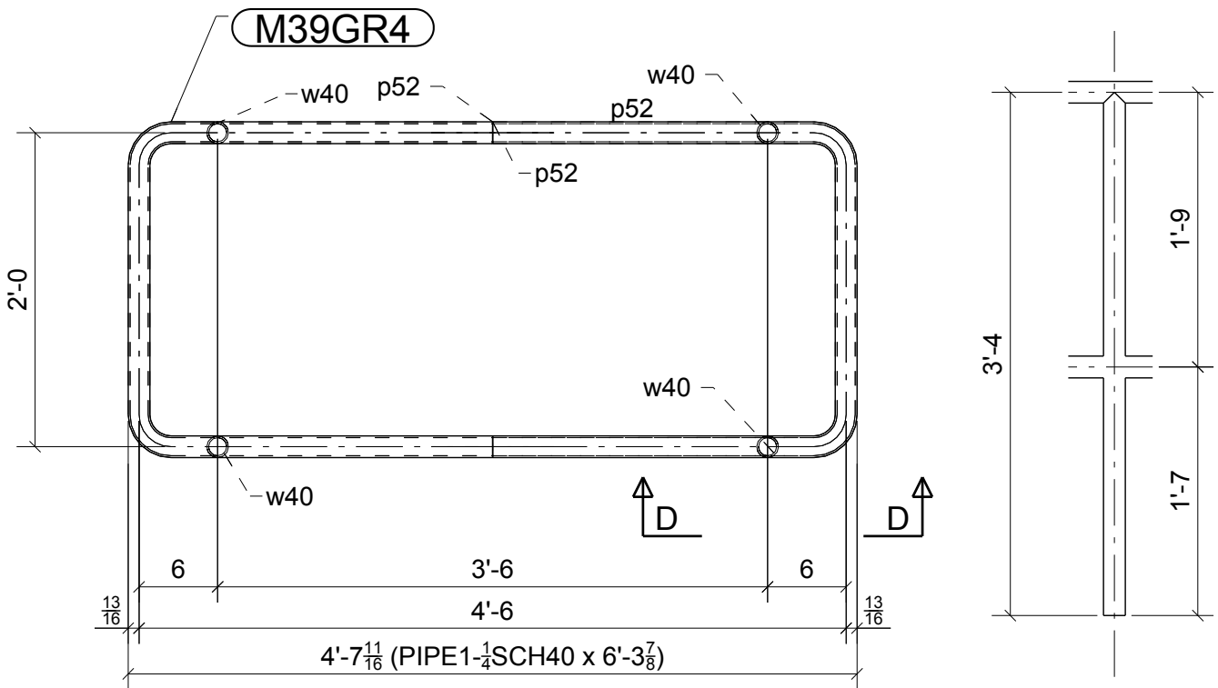
6 - GUARDRAILS - M39GR4
