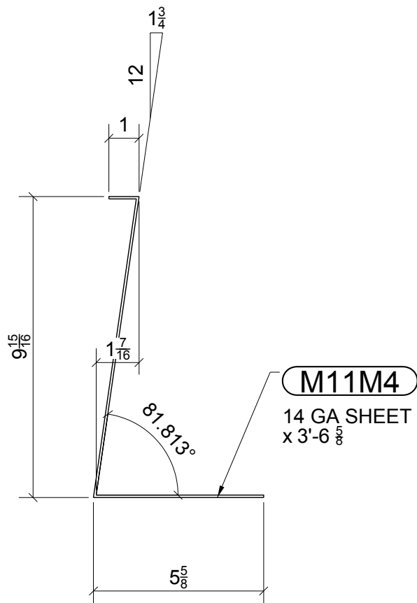
4 - TREADS - M11M4
