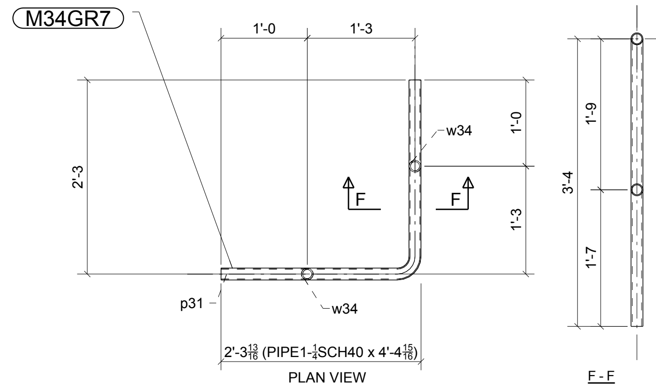
5 - GUARDRAILS - M34GR7
