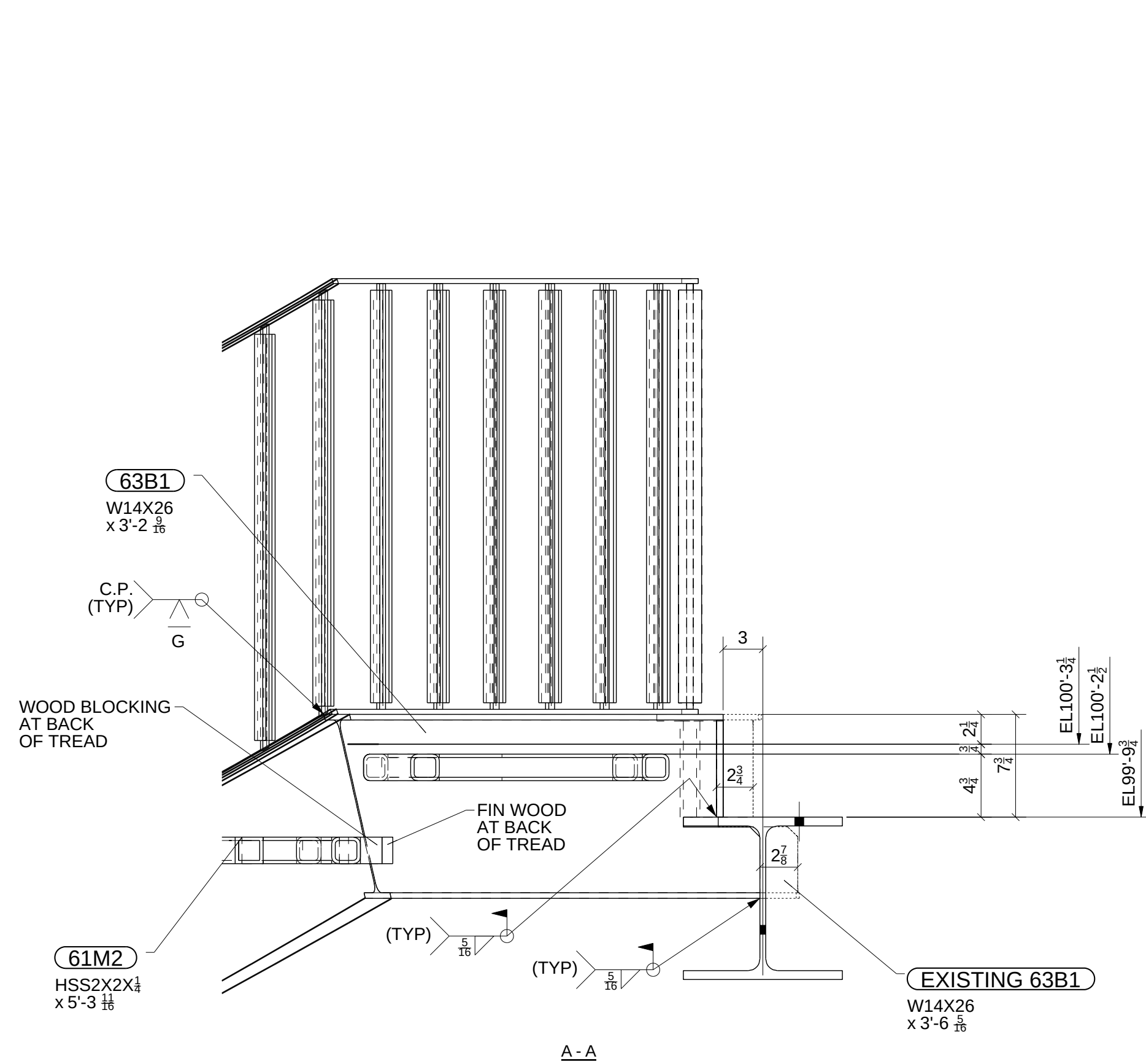
A-A
