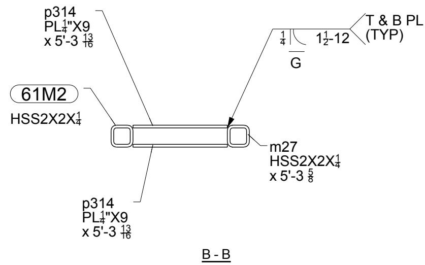
B - B
