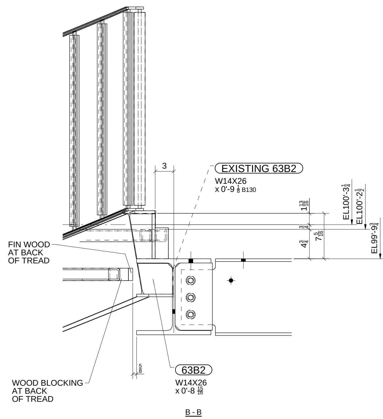
B-B
